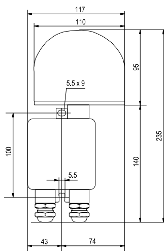
CEL-10-48-F dimensions
